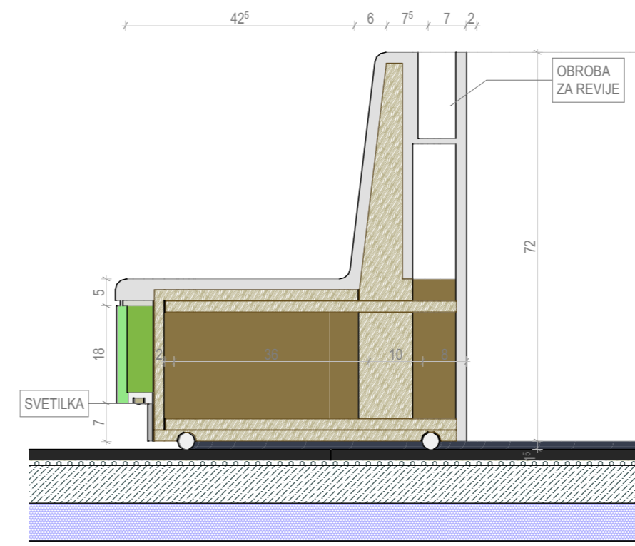
NO_RO_04 Prerez 1:10
